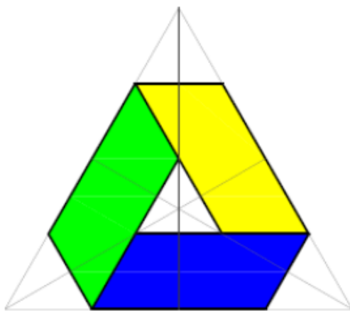
TRIANGOLO EQUILATERO DATO IL LATO
