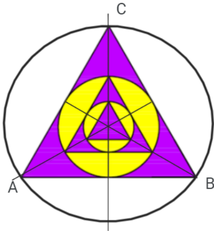
TRIANGOLO EQUILATERO DATA LA CIRCONFERENZA
